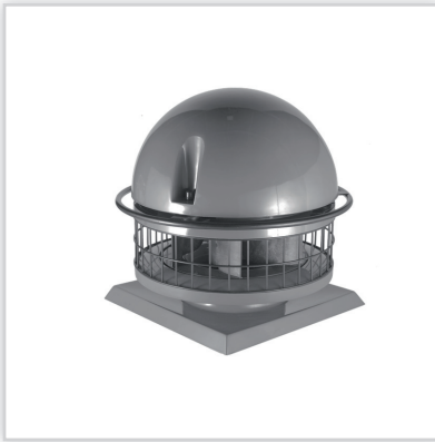
Wentylator dachowy DA (standard), DAK (kwasoodporny). Typ: DAs,(k)160, 200, 250, 315, 400, 500, 630 DAs(k)-P2 i P3 (dwu- i trójbiegowy) 200,250,315. Obroty [obr/min-1]: 700, 900, 1400, 2800 obr/min-1. Wydajność [m 3 /h]: 200-36000. Moc [kW]: 0,04/7,5. Napięcie [V]: 1 x 230 lub 3 x 400. Cisnienie akustyczne [dB(A)-(1 m)]: 51-89. Wykonanie: laminat poliestrowo-szkłany. Kolor: dowolny wg tabeli RAL. Cena netto [zł]: 1900-16 755.
